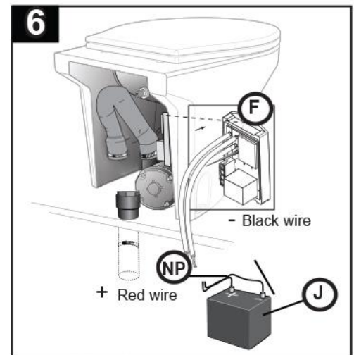
Conectar ⑥ a conector ⑦; luego a ⑧
