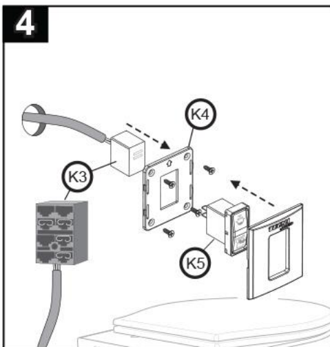
Pasar ③ a través de ④; conectar a ⑤; cubrir el orificio y avanzar K4 con los tornillos
