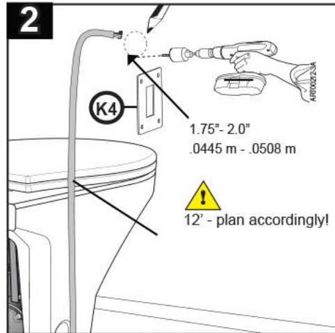
1. Marcar / hacer un orificio de 1.75 - 2.0 pulg. (4.5 - 5 cm) en la pared 2. Colocar ④ sobre el orificio; perforar los orificios de los tornillos
