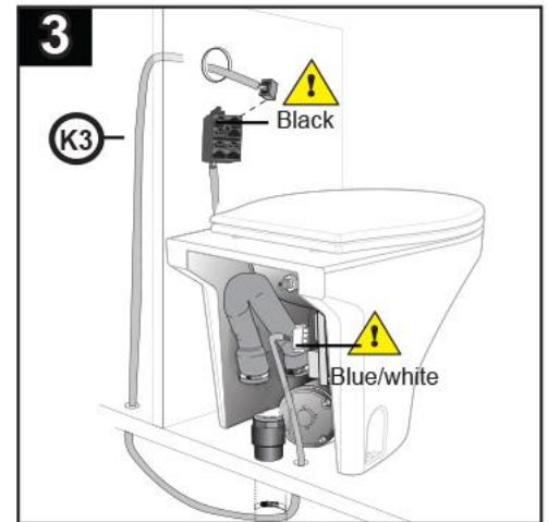
⚠ Colocar conectores; pasar ③ a través de la pared
