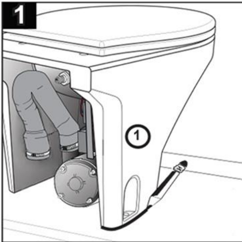
Colocar ① en posición permanente; trazar perímetro.
